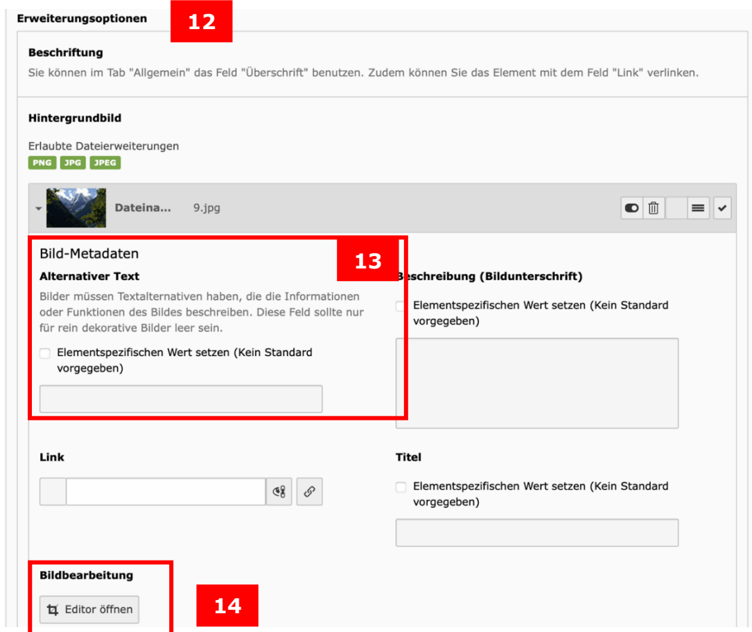
Abbildung 5: Bild-Metadaten ergänzen
