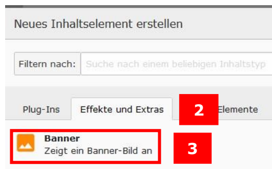
Abbildung 3: Banner-Bild einfügen
